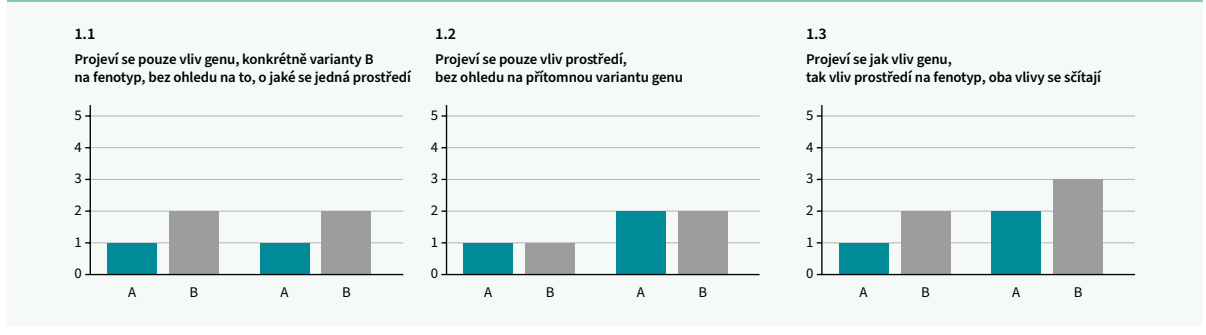
Graf 2 | Možné vztahy mezi dvěma faktory na fenotyp. Vztahy jsou zde nelineární, různými způsoby spolu interagují. Jako faktor na ose X je použit gen (dvě alely, „A“ a „B“) a na ose Y prostředí (protektivní působení znázorněno zeleně a rizikové šedě).
