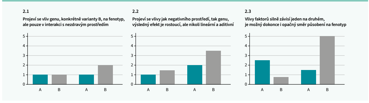
Graf 2 | Možné vztahy mezi dvěma faktory na fenotyp. Vztahy jsou zde nelineární, různými způsoby spolu interagují. Jako faktor na ose X je použit gen (dvě alely, „A“ a „B“) a na ose Y prostředí (protektivní působení znázorněno zeleně a rizikové šedě).
