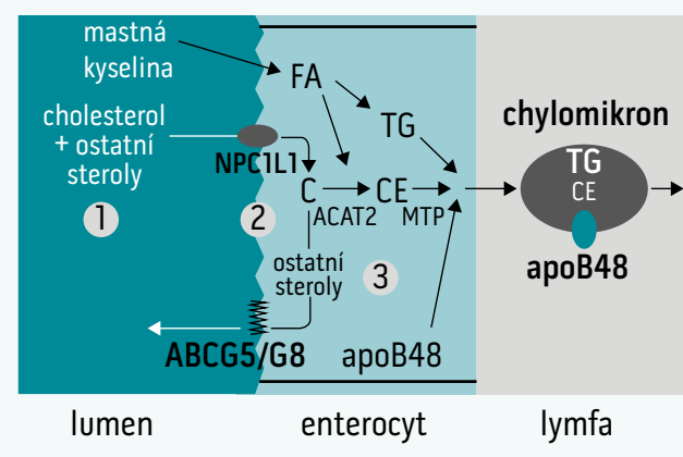
Schéma 1. Metabolismus fytosterolů – inkorporace do micel (1), absorpce (2) a intracelulární esterifikace (3). Upraveno podle [4]
